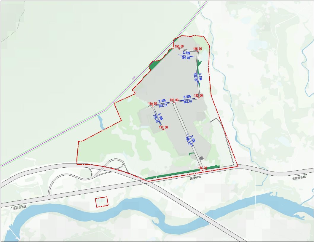
道路竖向规划图
