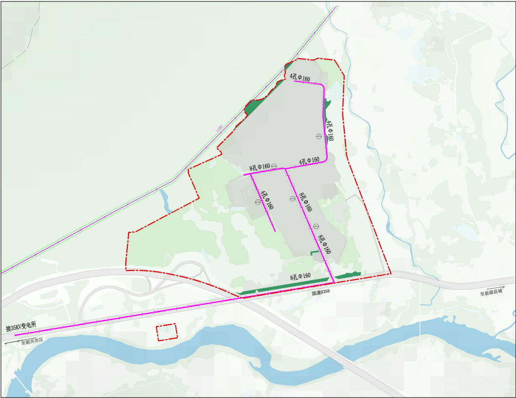
电力工程规划图
